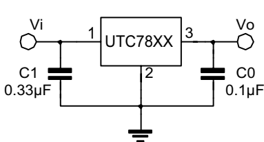
图1 测直流电参数电路图
