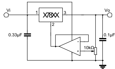
图7 可调型稳压电路
